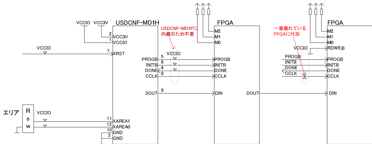
図 5.1.3 USDCNF-MD1H-001A 接続例
