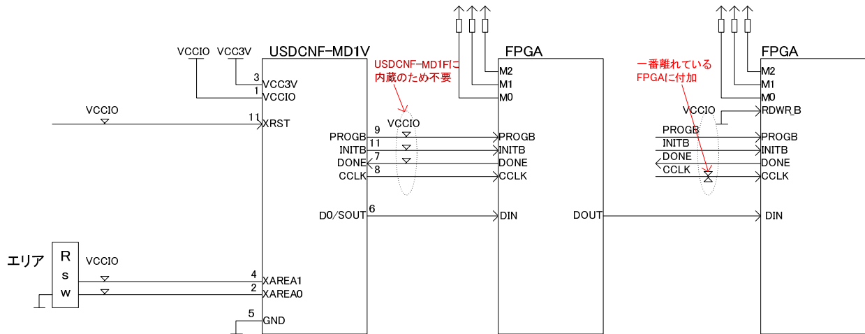
図 5.1.2 USDCNF-MD1V-001A 接続例
