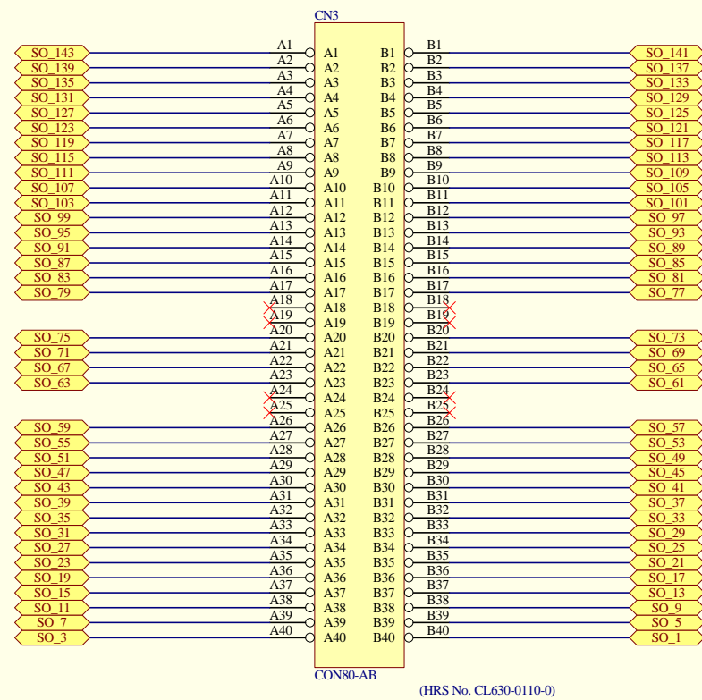
SODIMM Top Layer
