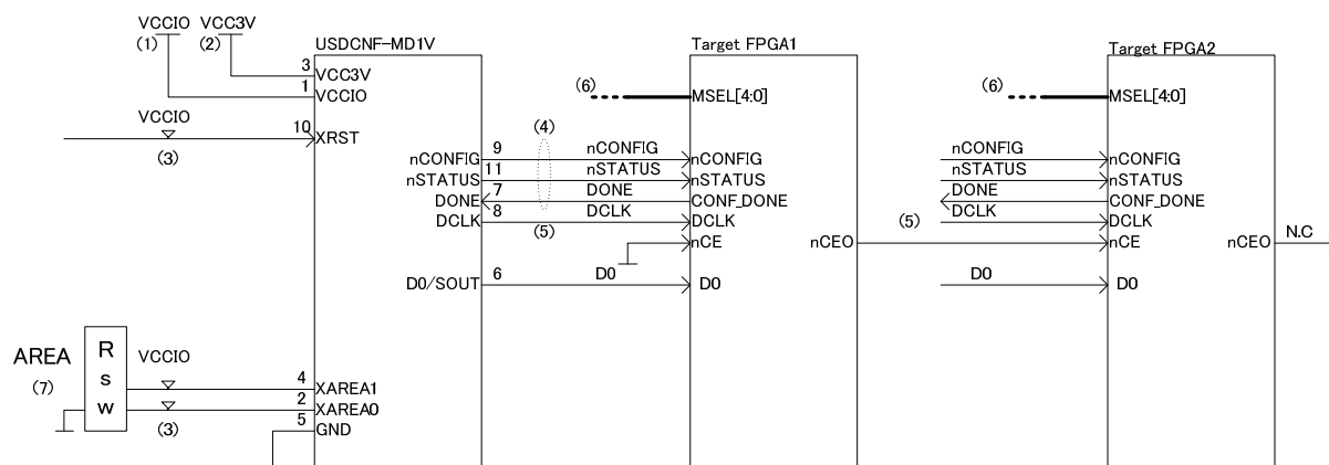
図 5.2 USDCNF-MD1V-001A 接続例
