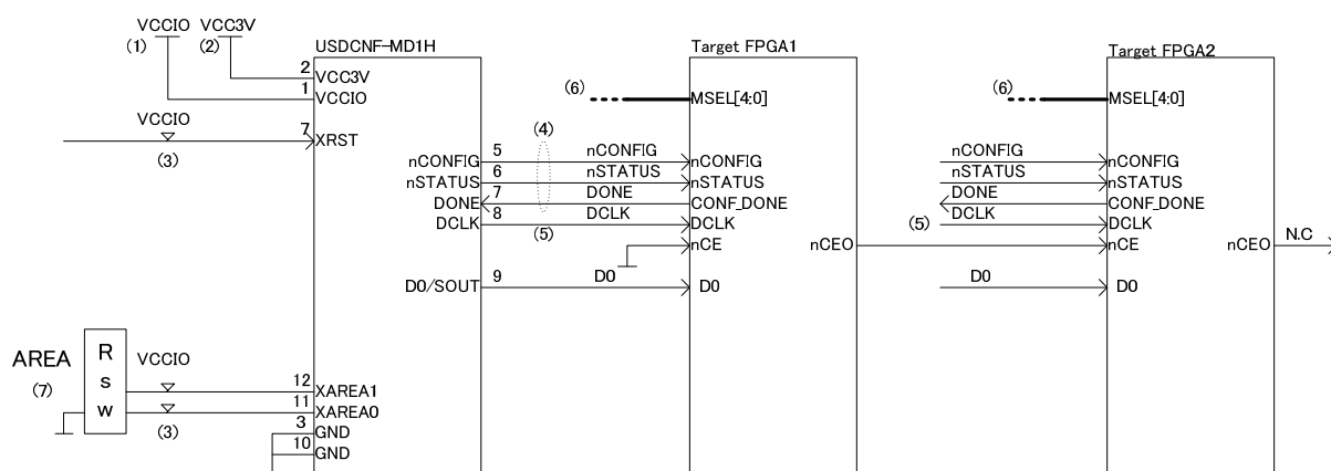
図 5.3 USDCNF-MD1H-001A 接続例
