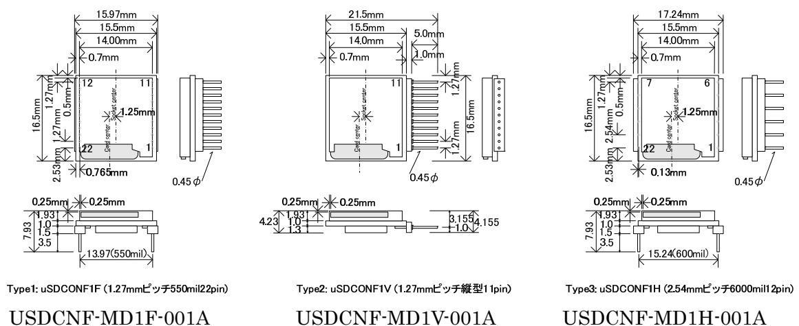
図 2.1 uSDCONF1 形状図
