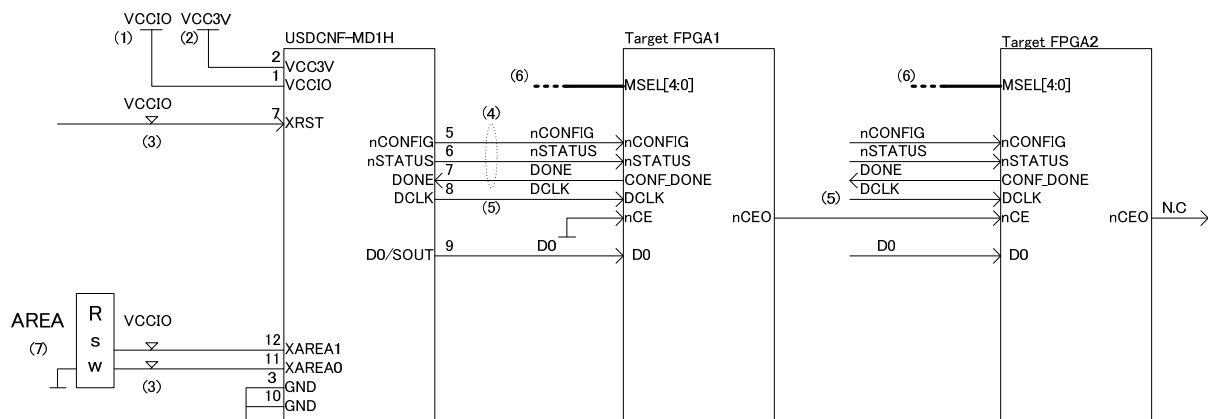
図 5.3 USDCNF-MD1H-001A 接続例
