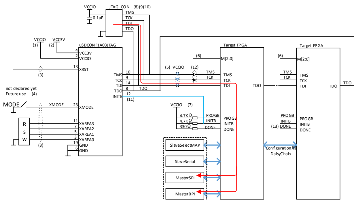
図 6.1.3 uSDCONF1A03JTAG その他のコンフィグレーションモードとの併用接続例
