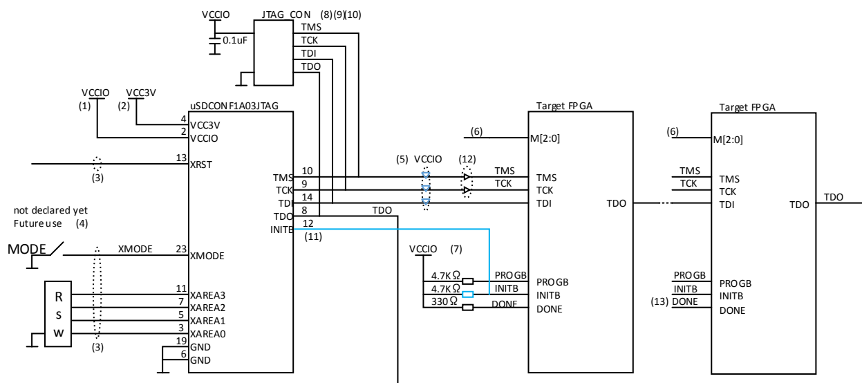
図 6.1.2 uSDCONF1A03JTAG Daisy Chain 接続例
