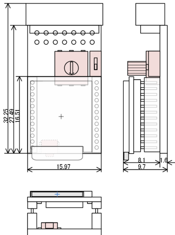
図 3.1 59JTagStick 形状図
