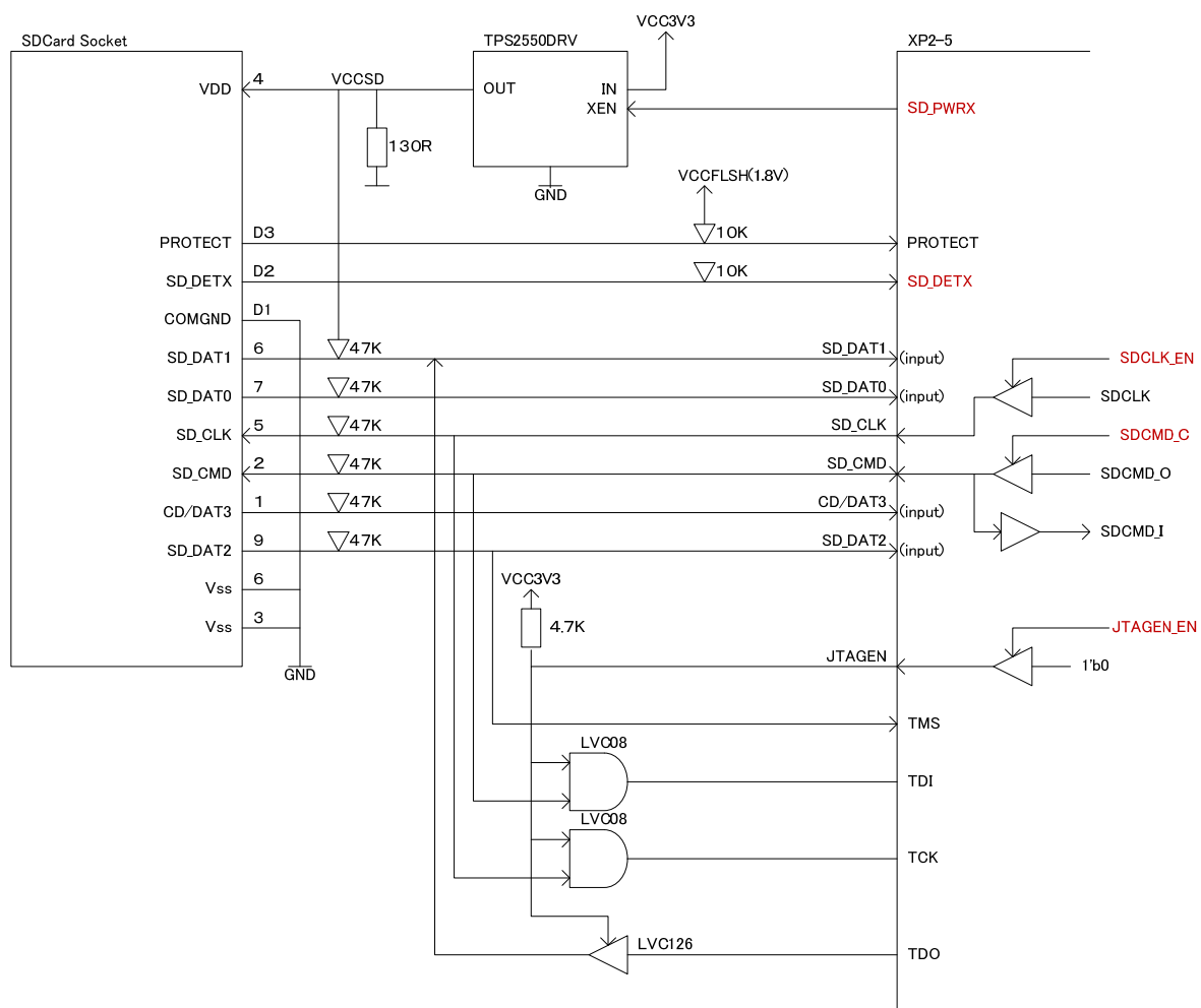
図 9.2.1 SDCard インタフェース部構成図
