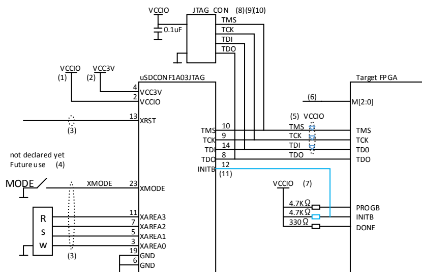
図 5.1.1 uSDCONF1A03JTAG 1:1 接続例
