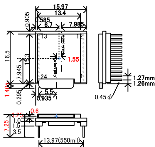
図 3.2 uSDCONF1A03JTAG 形状図
