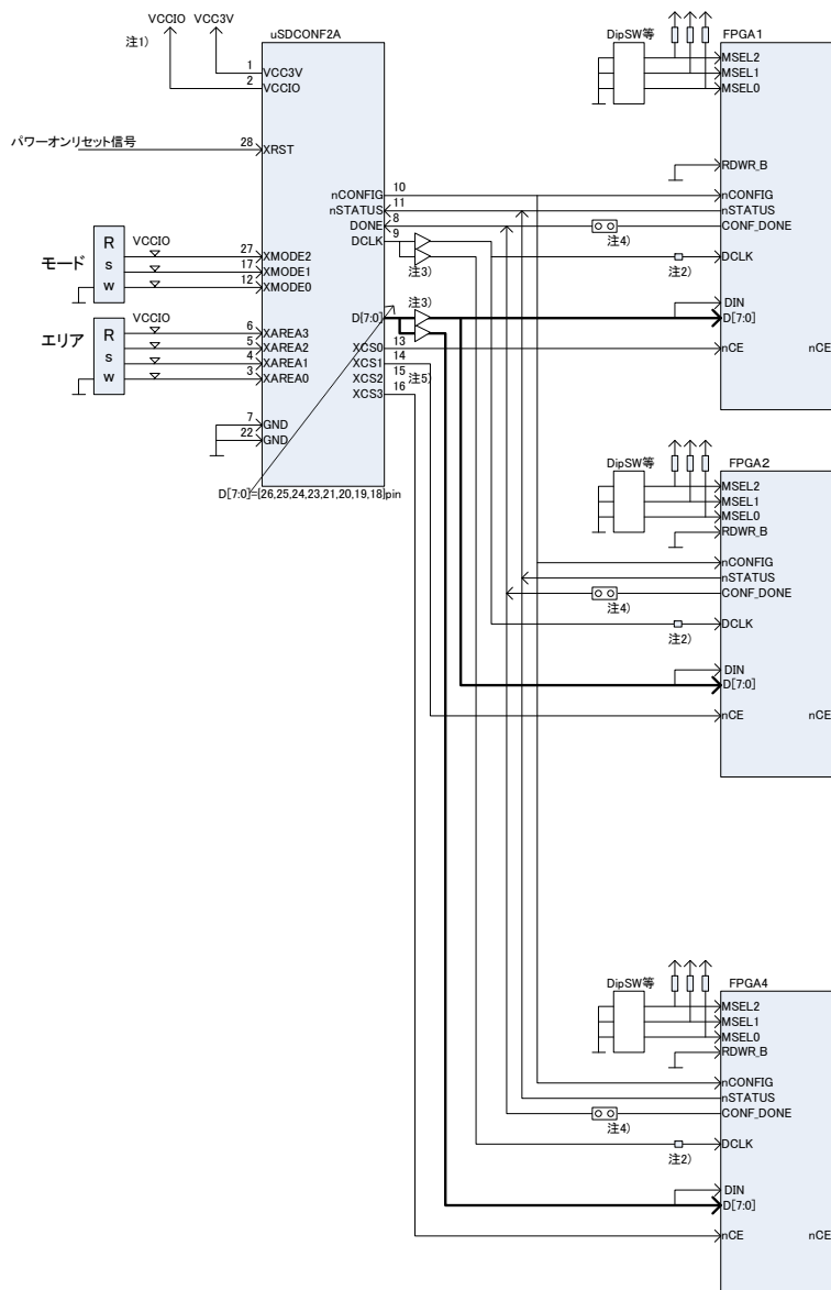
図 5.1.2.1 PS/FPP8 接続例(1:N 接続)
