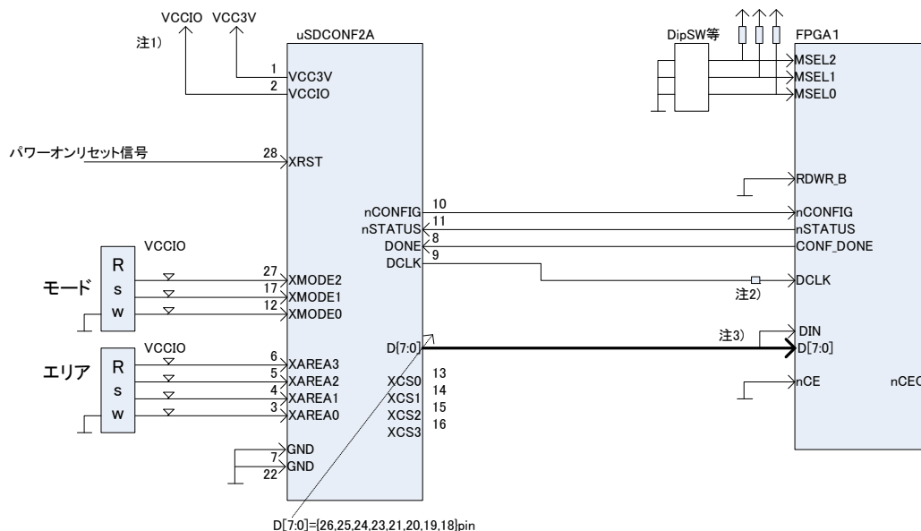
図 5.1.1.1(1) PS/FPP8 接続例(1:1 接続)
