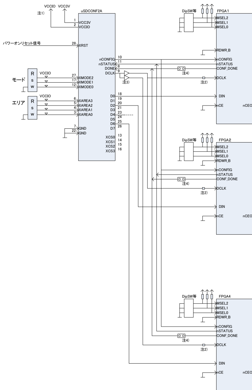
図 5.1.3.2 bit 多重方式による Multi-FPGA 接続例(4 多重)
