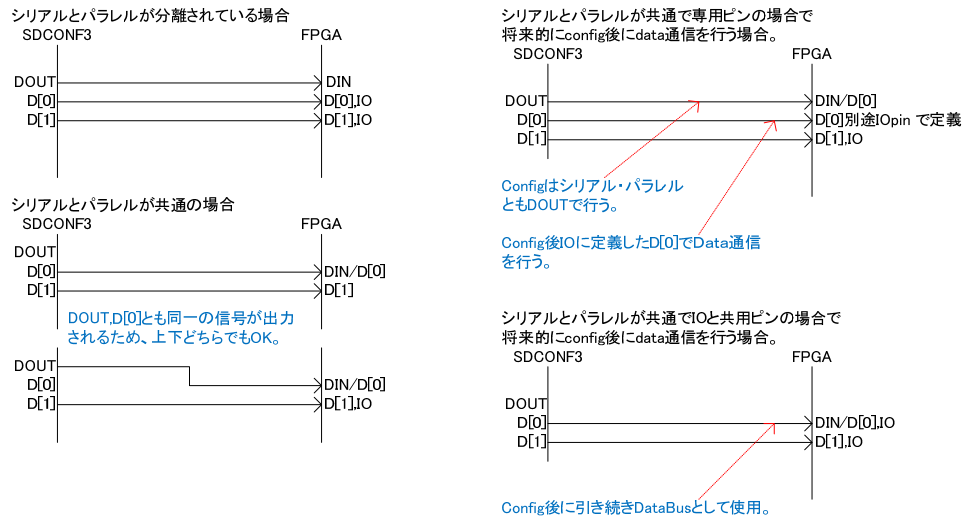
図 5.1.1.1(3) DOUT/D[0]接続イメージ
