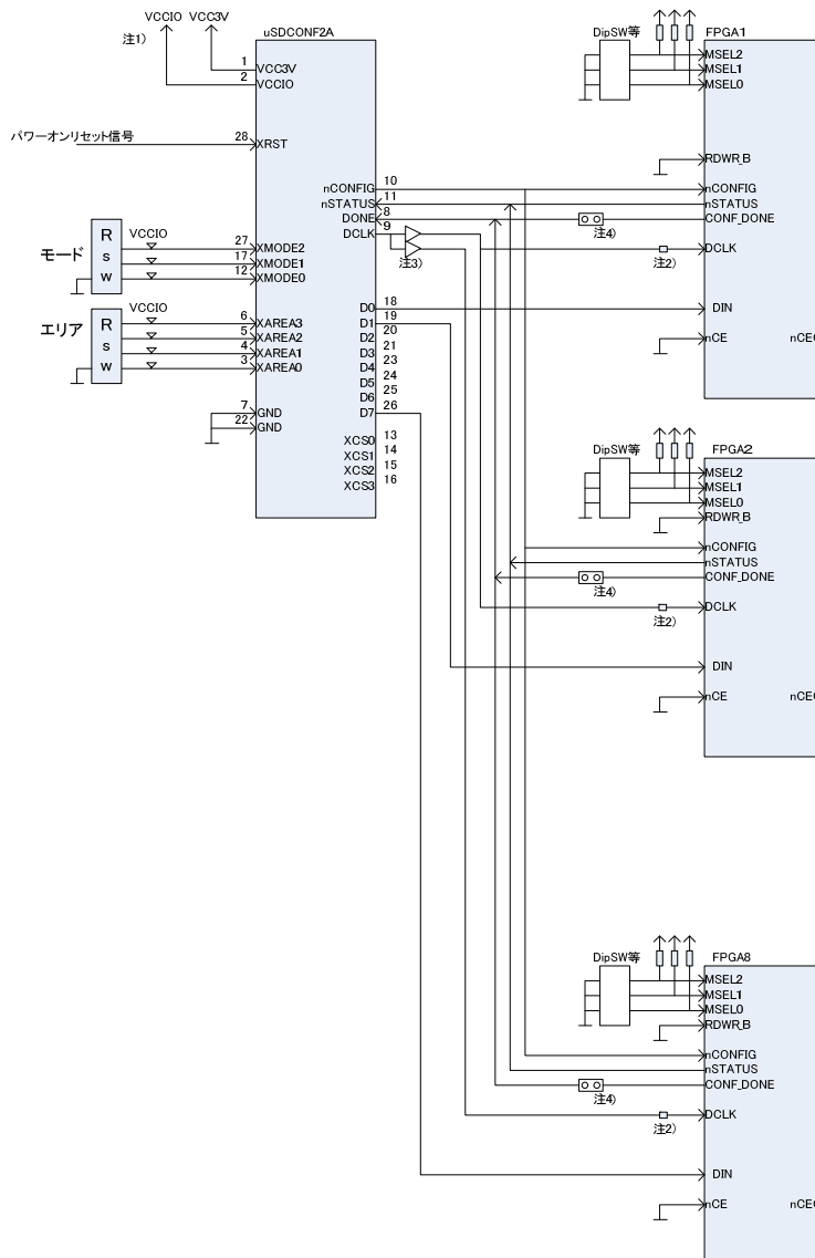
図 5.1.3.1 bit 多重方式による Multi-FPGA 接続例(8 多重)
