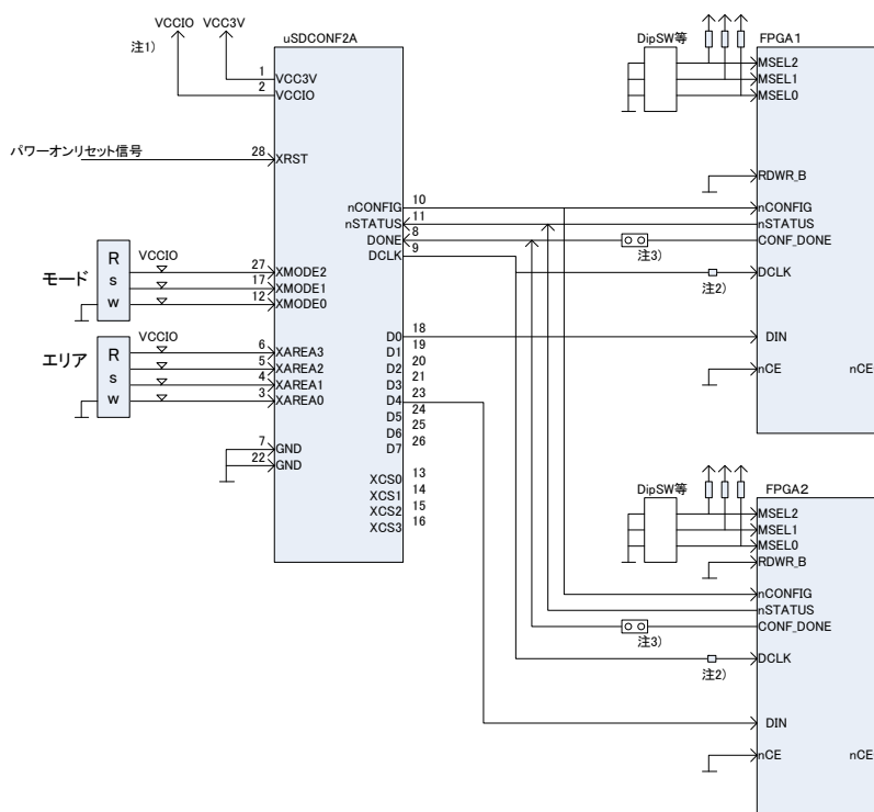
図 5.1.3.3 bit 多重方式による Multi-FPGA 接続例(2 多重)
